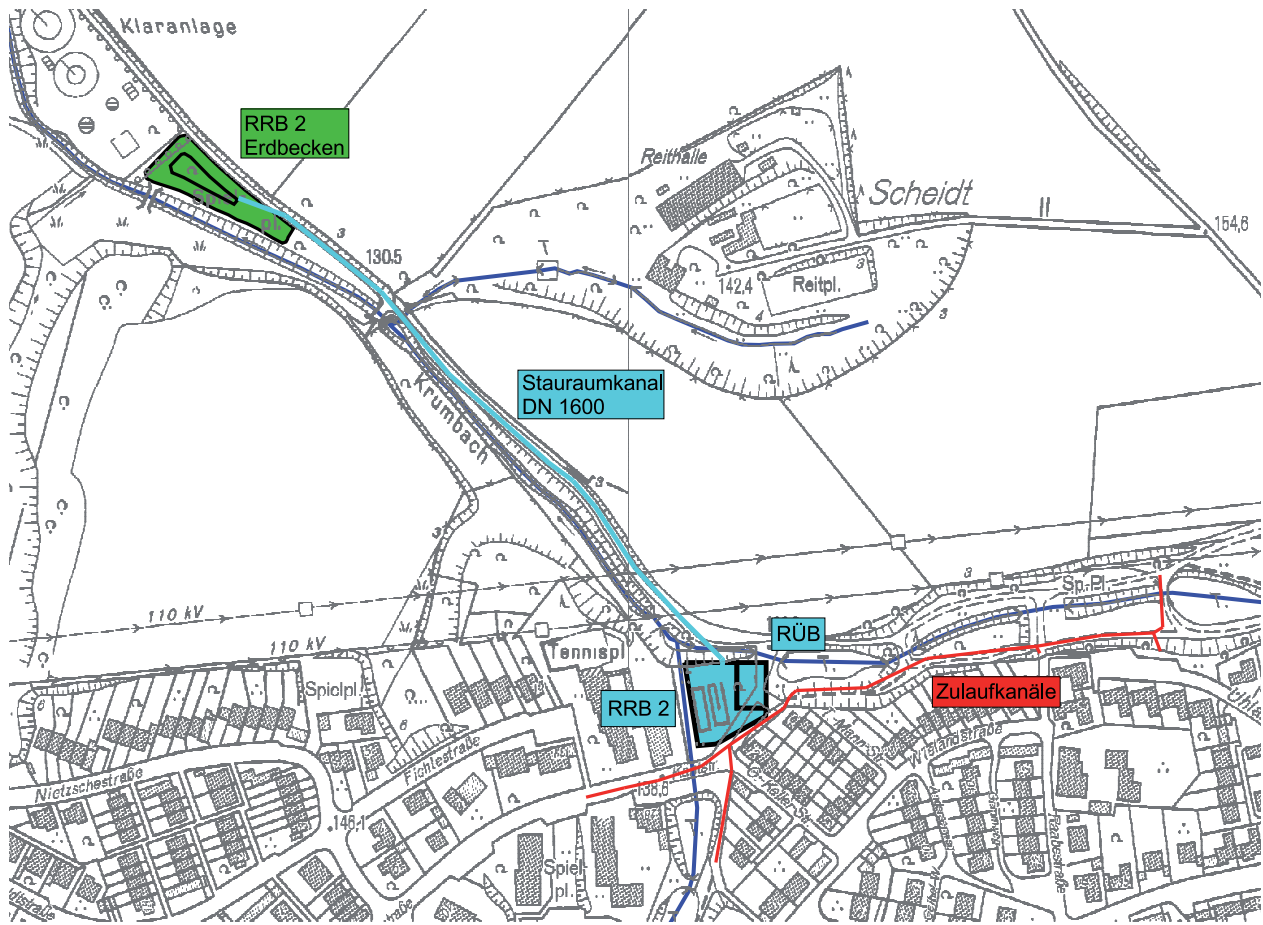
Lageplan Neubau der Regenbeckenanlage Kantstraße
