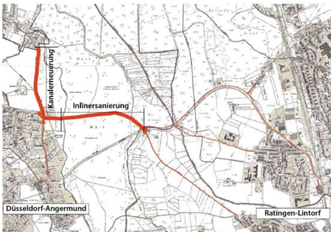
Übersichtsplan Abwassersammler Ratingen-Lintorf und Düsseldorf-Angermund
