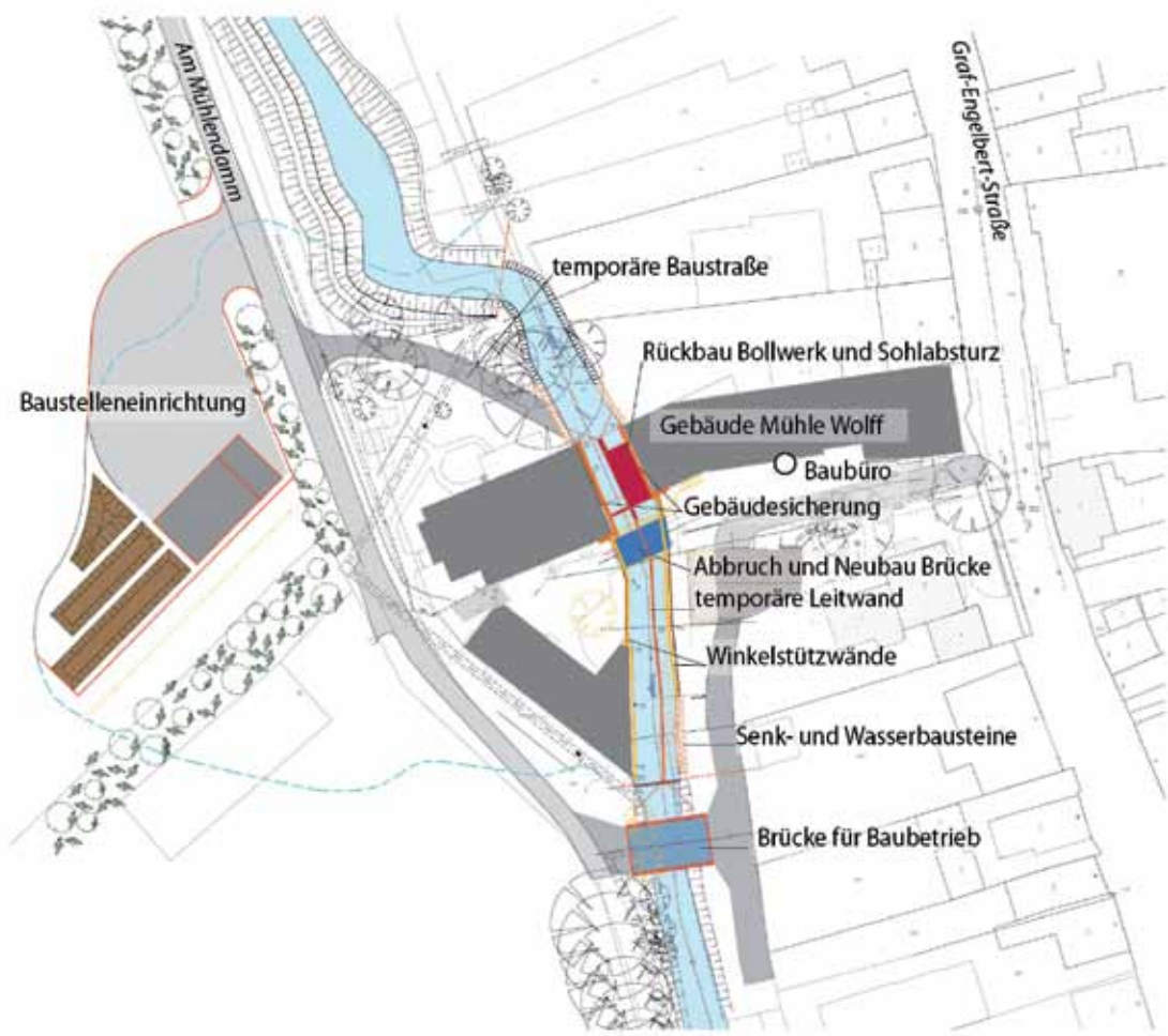
Lageplan Baumaßnahme an der Anger Bereich „Mühle Wolff“
